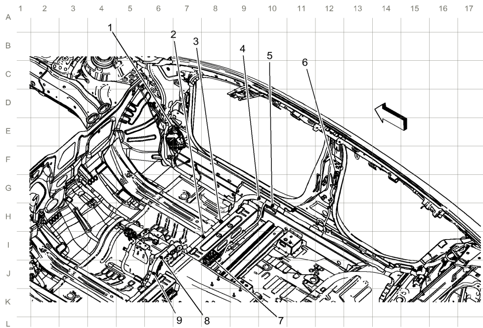
车身线束布线 - 乘客舱右侧
